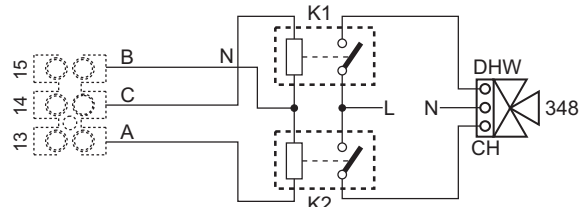
рис. 96- Подключение 3-х ходового клапана с 3 проводами
