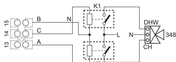
fig. 96- Raccordement de la vanne 3 voies à 3 fils
