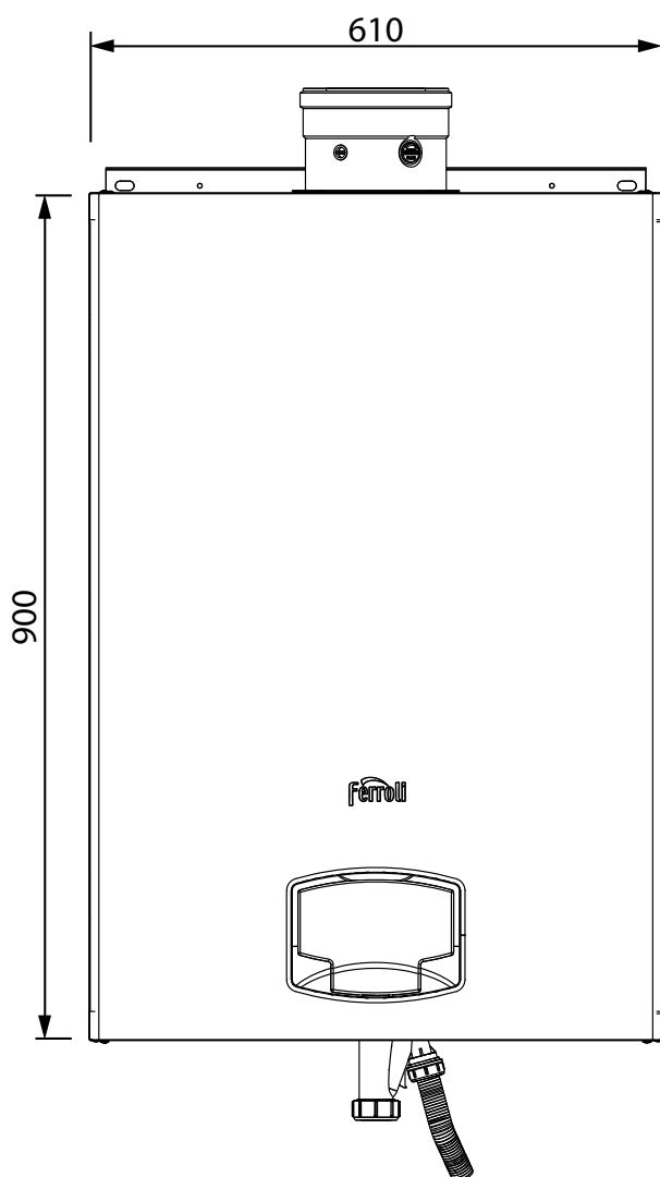
рис. 84- Вид спереди
