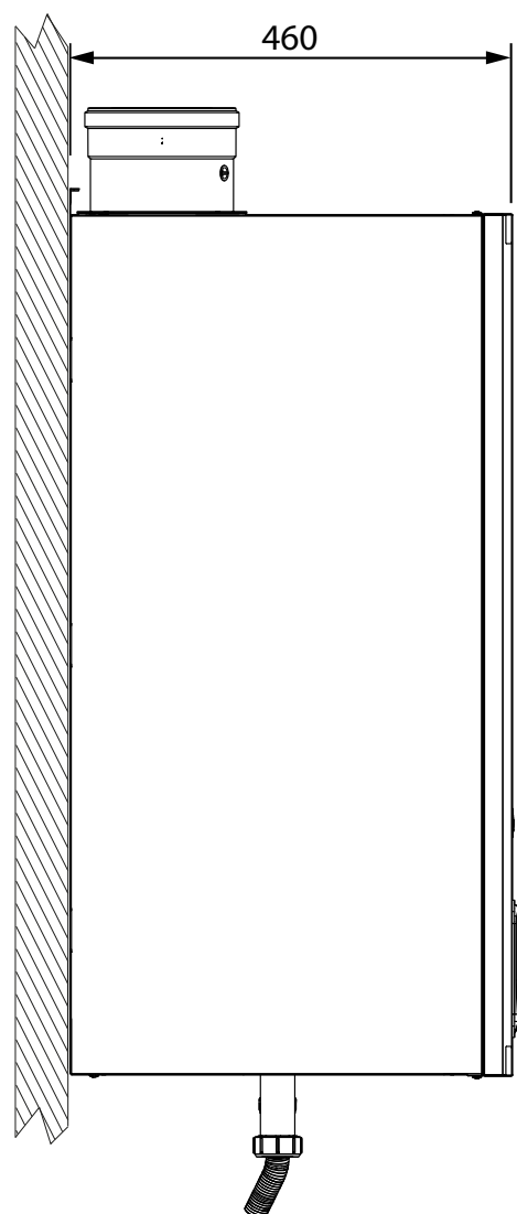
fig. 85- Vue latérale
