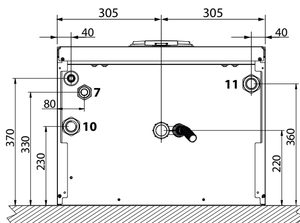
рис. 87- Вид снизу
