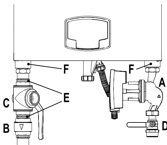
fig. 34- Caldera con kits instalados
