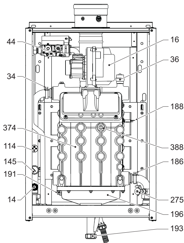
fig. 89- Vue générale mod. TORO W 99 et TORO W 120
