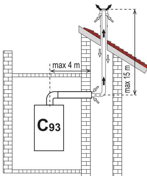
fig. 62- Exemples de raccordement aux conduits de fumées (⇨ = Air / ⇨ = Fumées)
