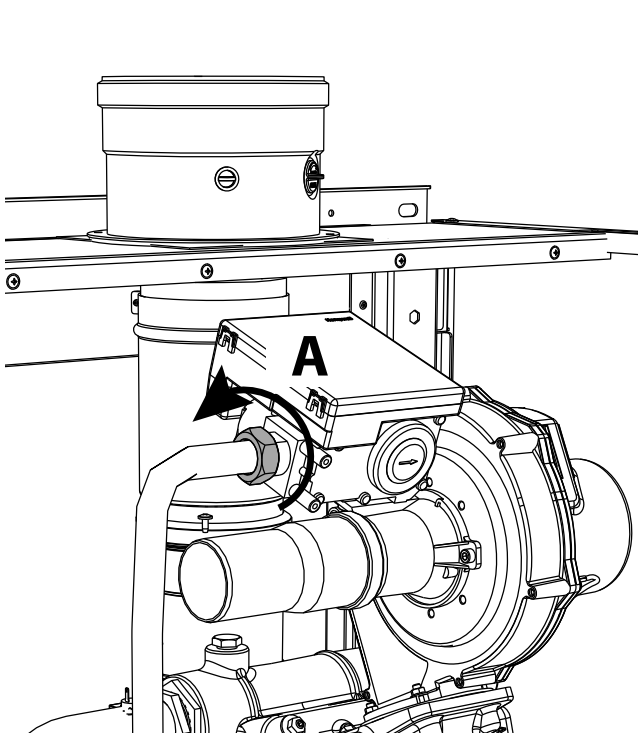
fig. 68- Modèles W 60 et W 80
