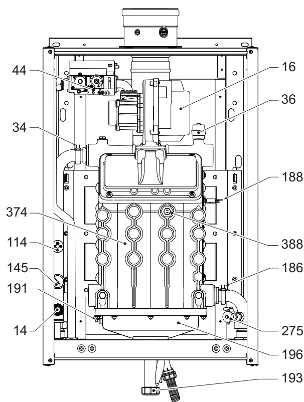
fig. 89 - Vista generale mod. TORO W 99 e TORO W 120
