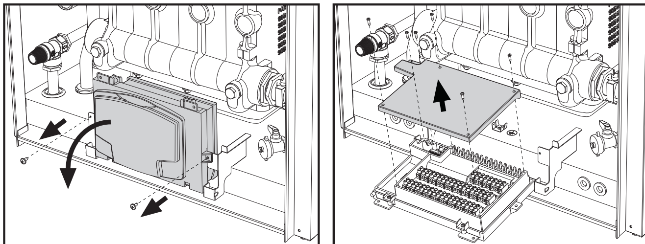
fig. 52 - Morsettiera elettrica
