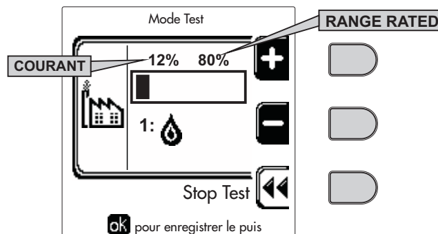
fig. 80- Mode TEST (exemple puissance de chauffage = 80%)
