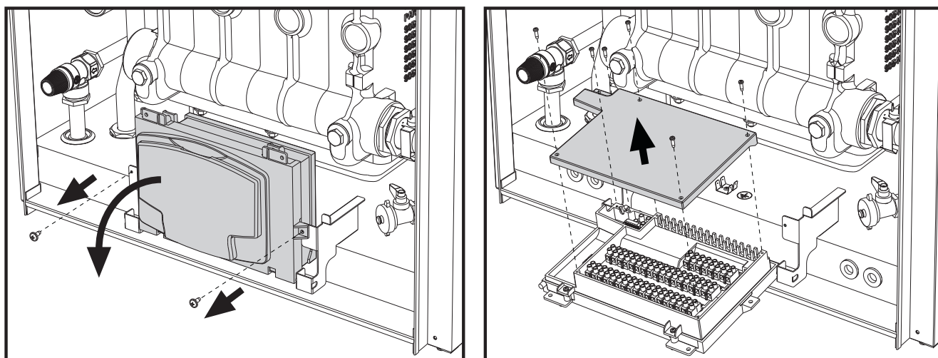
fig. 52- Bornier électrique
