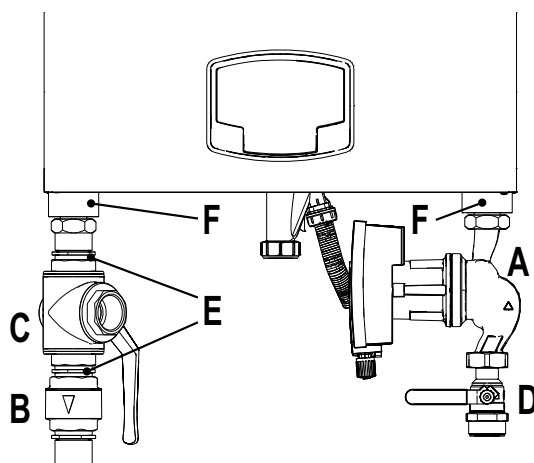
fig. 34- Chaudière avec les kits installés
